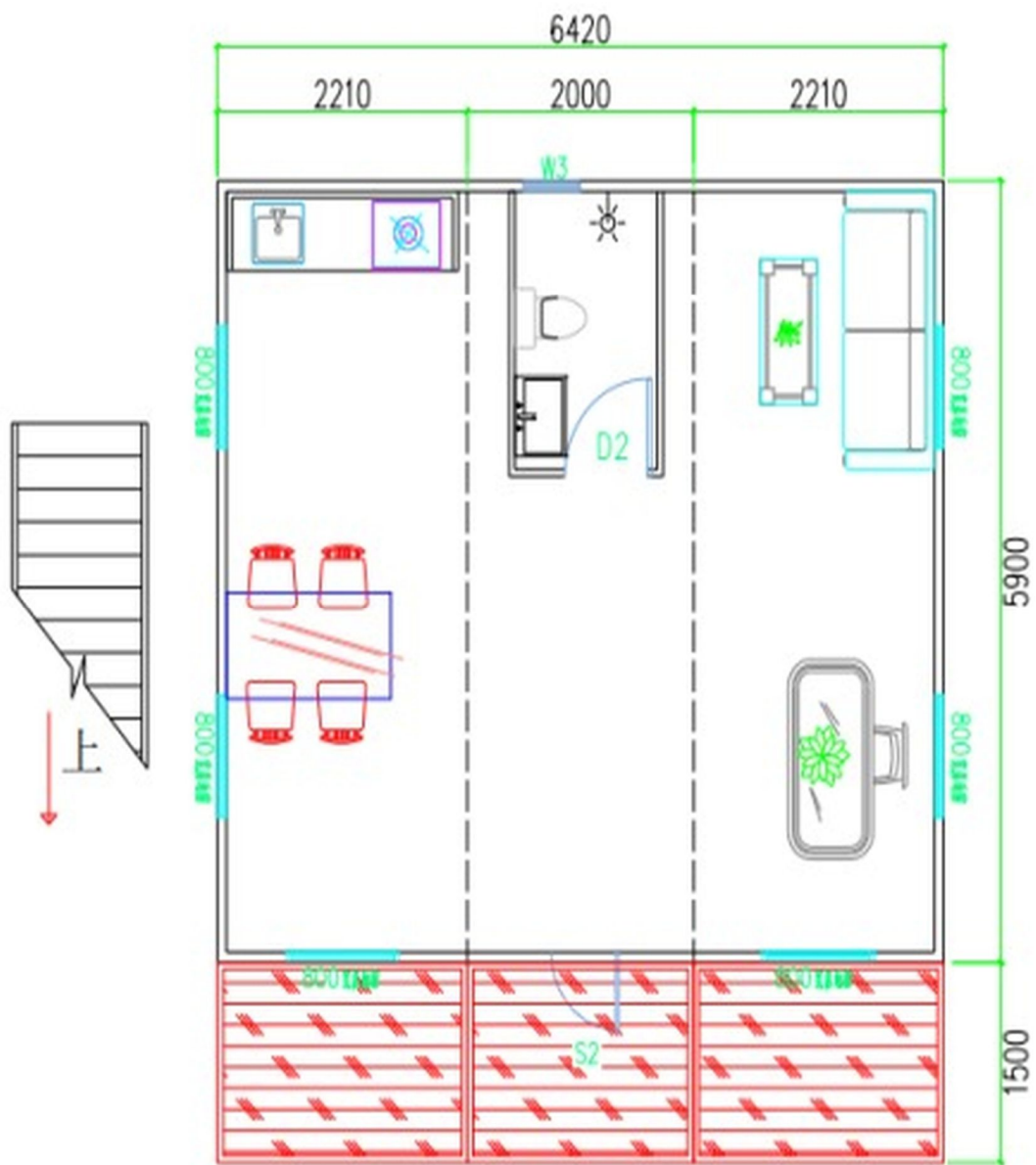
一层平面布置图
