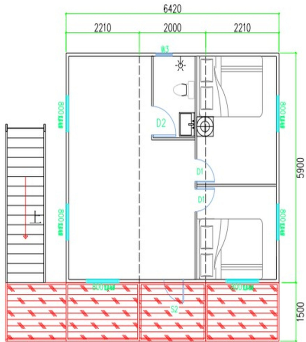
二层平面布置图
